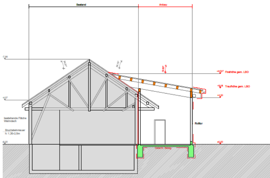
Schnitt D-D
