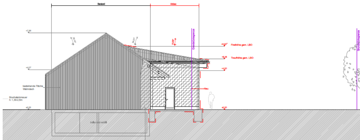
Ansicht West
