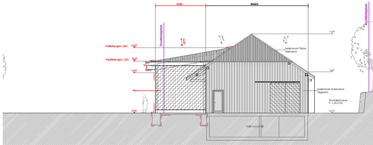
Ansicht Ost
